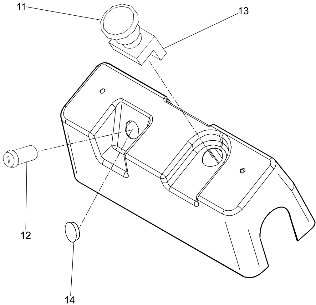
5310-057 Start/stop switch [2000-07-03] Start/stopströmställare; Schalter Fahren/Anhalten; Interrupteur (coupe-circuit) démarrage/arrêt
