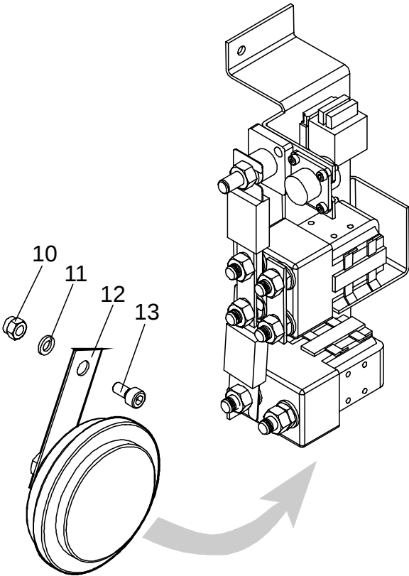
5160-032 General alarm signals (audible/visual) [1999-11-24] Signal/larm (ljud-/ljus-); Warn-/Alarmsignale (Aukust./Opt.); Avertisseur (sonore/lumineux), dispositifs d'alarme
